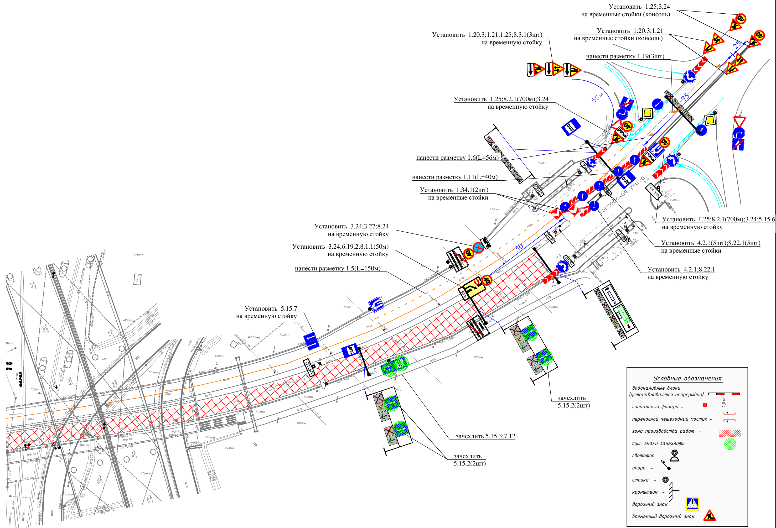
Схема ОДД на период производства работ (этап 3)
